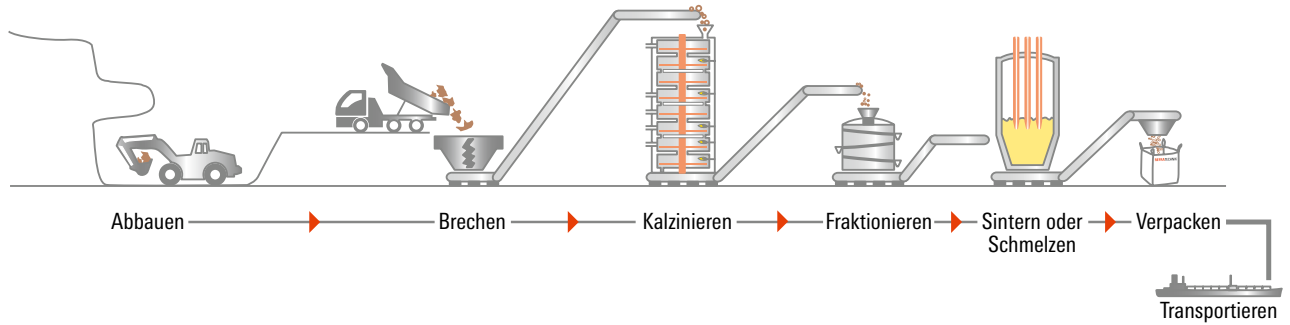
Beispiel: Weiterverarbeitung Zementindustrie
