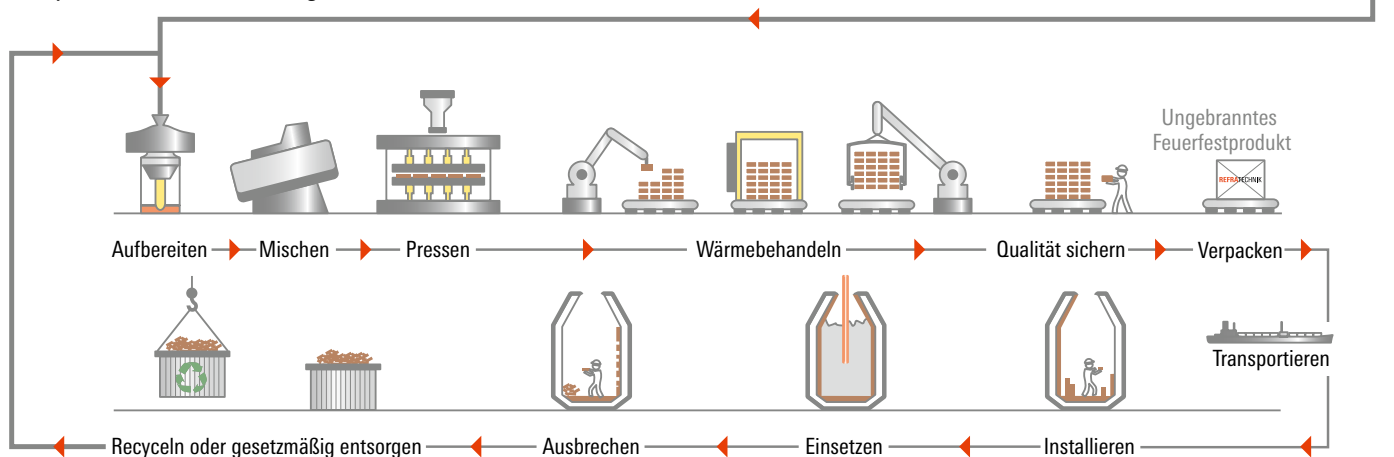
Beispiel: Weiterverarbeitung Stahlindustrie
