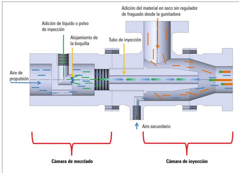
Gráfico 1: Estructura/Principio de funcionamiento de la boquilla REFRAJET® Addmix
