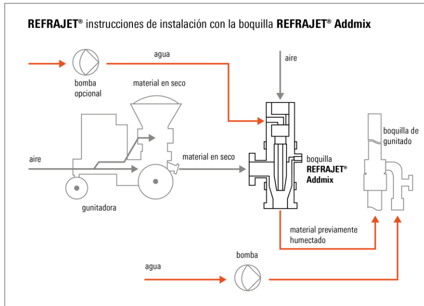
Gráfico 3: Uso de la boquilla REFRAJET® Addmix para hormigones de gunitado en seco de los tipos REFRAJET® regular, MC, LC, Hydrobond, Claybond, MW, LW, NC así como REFRASPECIAL® y REFRASPECIAL® CBP
