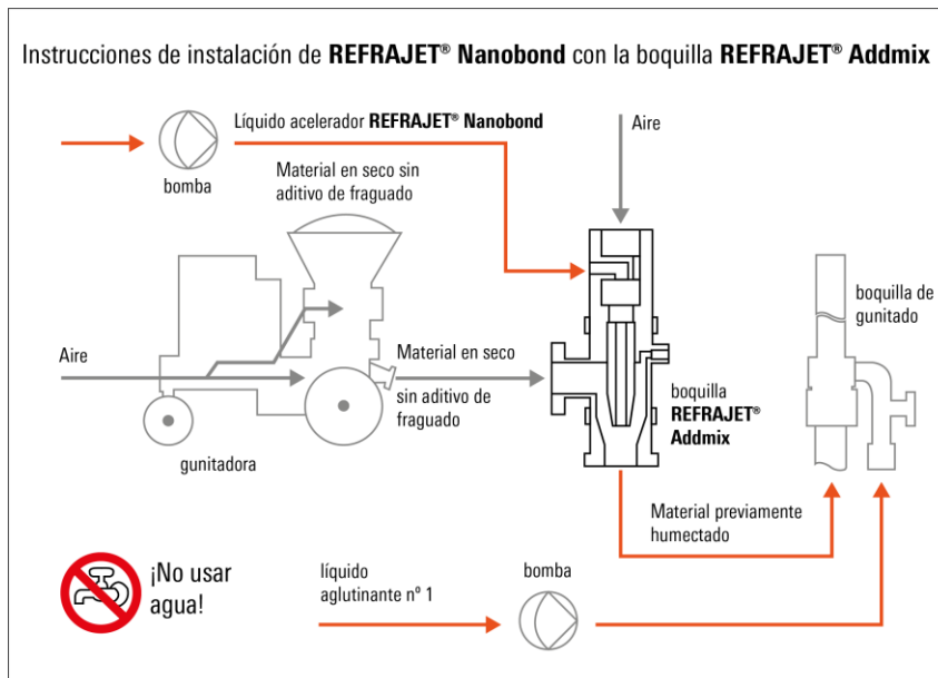
Gráfico 4: Uso de la boquilla REFRAJET® Addmix para hormigones de gunitado en seco del tipo REFRAJET® Nanobond El uso y el manejo de la boquilla REFRAJET® Addmix en combinación con el tipo de material REFRAJET® Nanobond se describe detalladamente en una norma de utilización (V 3.6) separada.
