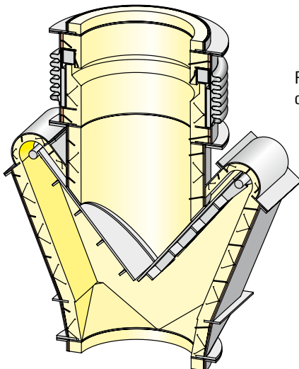
Soupape à clapet
