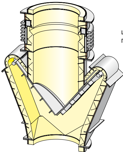
регулирующая заслонка
