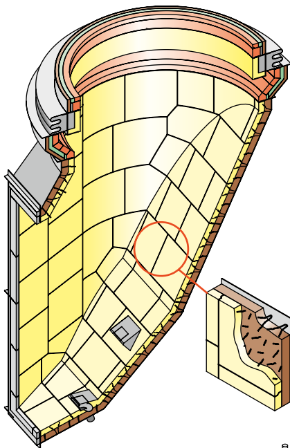
колено
