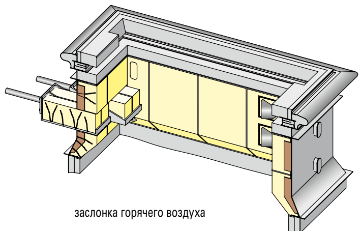
шиберный затвор люка газохода третичного воздуха
